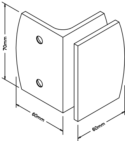
FIJA PARED-VIDRIO 90° 041224 (6481)
