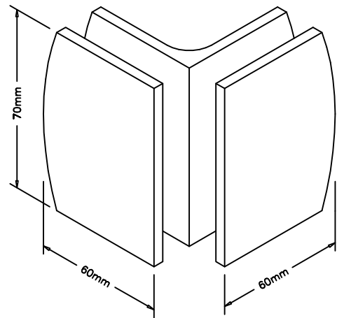
FIJA VIDRIO-VIDRIO 90° 041225 (6483)
