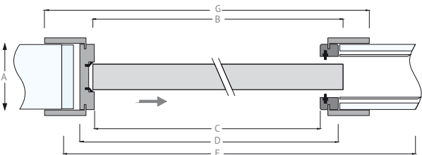
Sezione orizzontale Horizontal section Section horizontale
