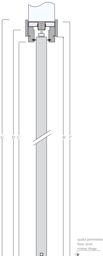
Sezione verticale Vertical section Section vertical
