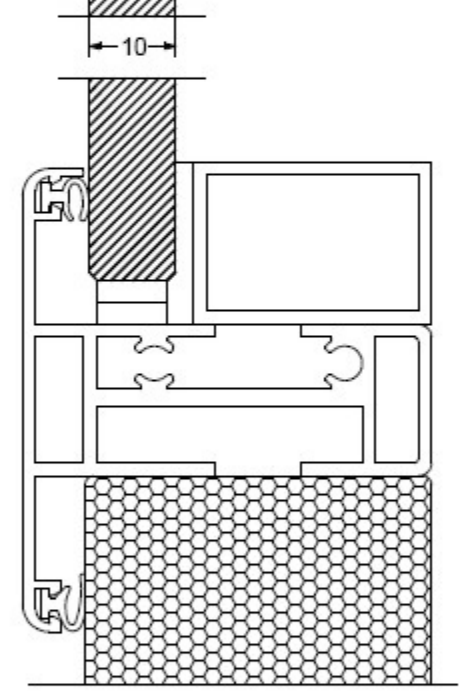
PARTICOLARE B
