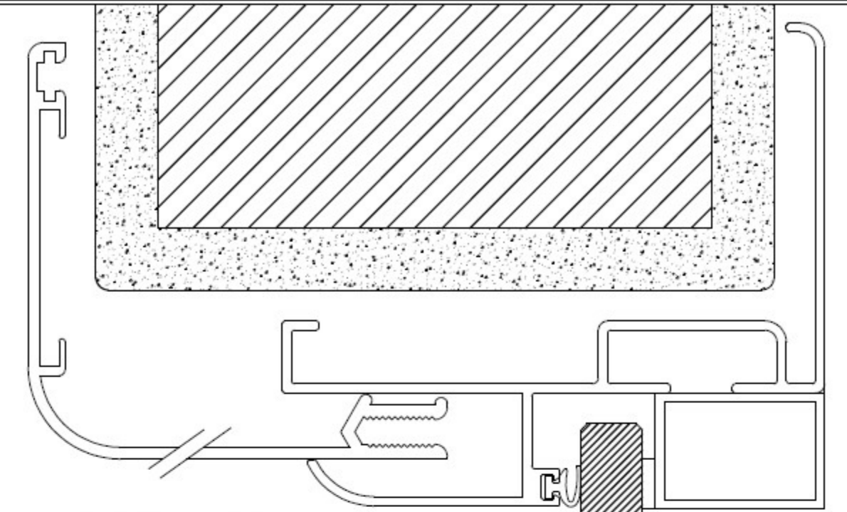
PARTICOLARE A
