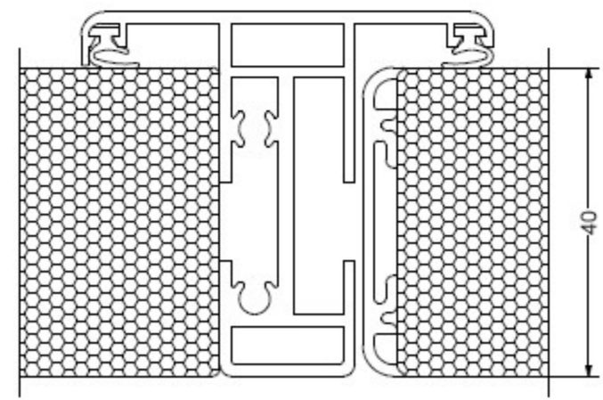
PARTICOLARE D
