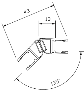
CIERRE MAGNETICO 135° 060366 POSITIVO 060367 NEGATIVO
