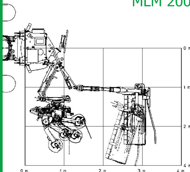
Rækkeviddediagram MLM 200
