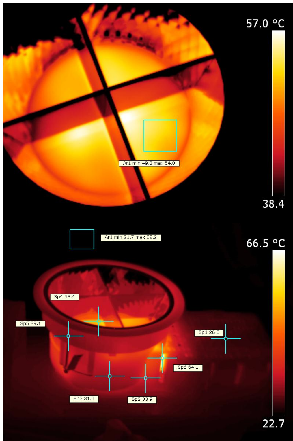
Warmtebeelden van de voorkant en de zijkant van de lamp.
