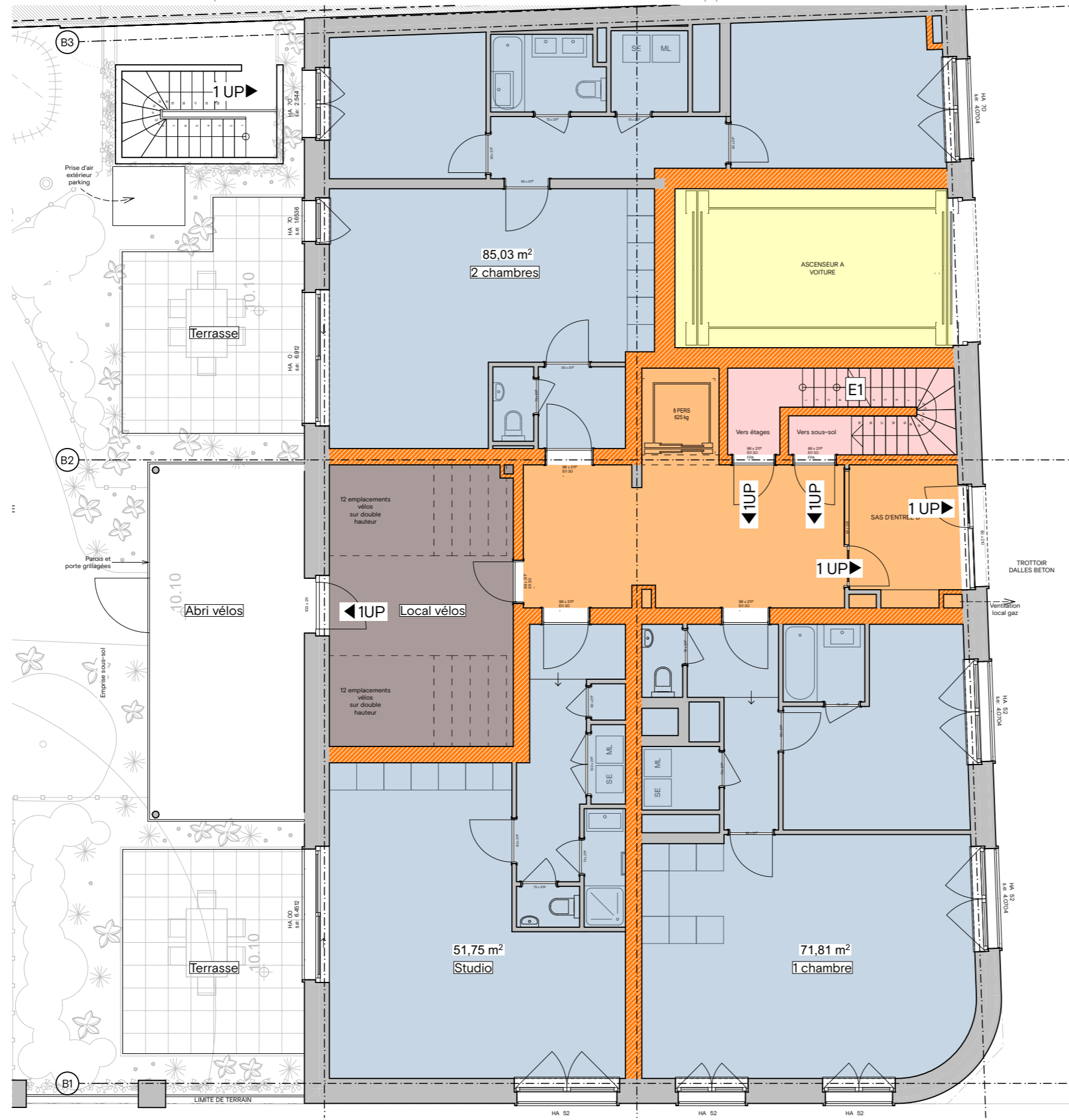
Bloc B - Plan rez-de-chaussée Plans de compartimentage
