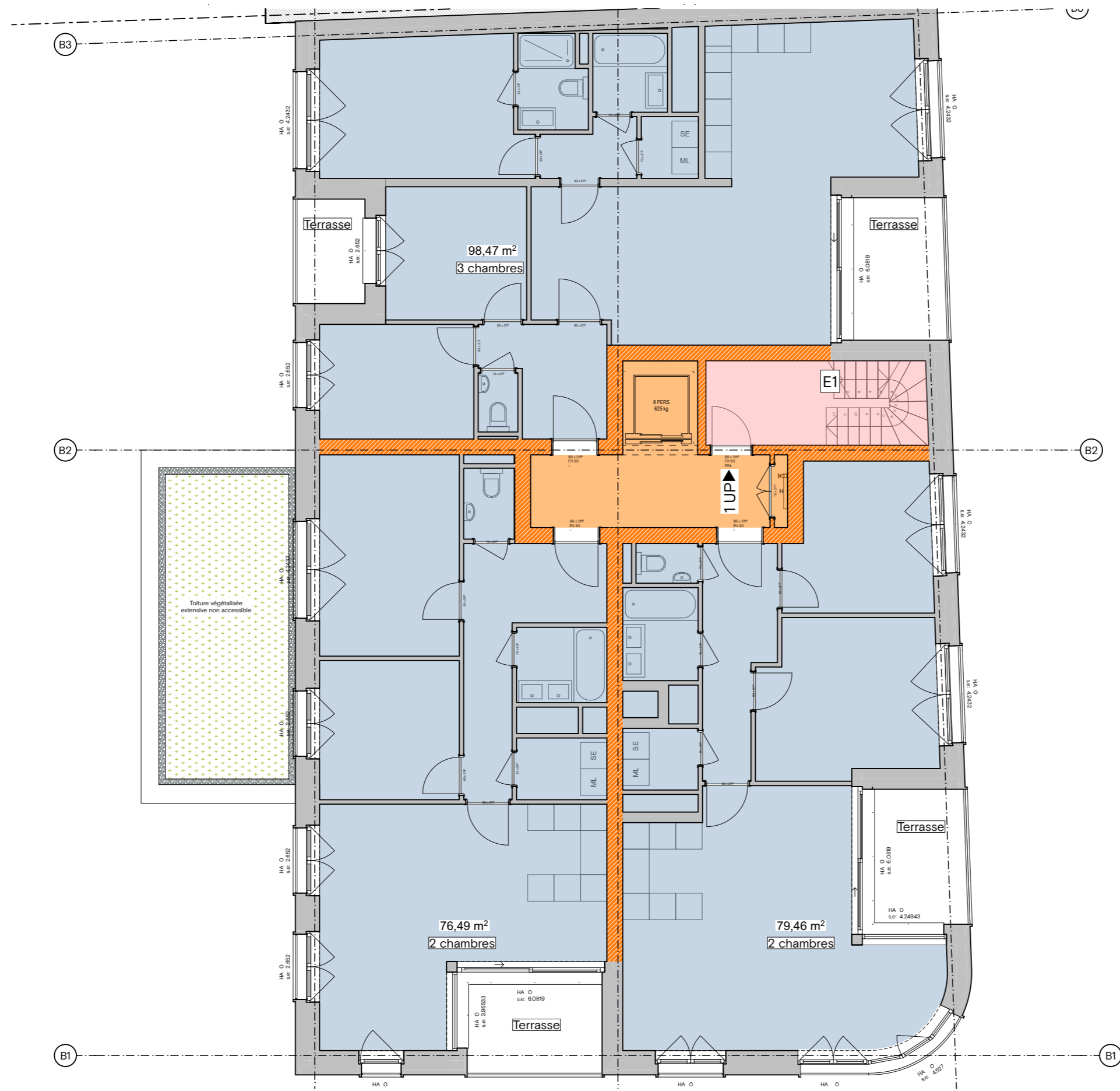
Bloc B - Plan étage type (+1 +2 +3 +4 +5)
