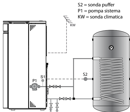
fig. 11 - Configurazione con puffer
