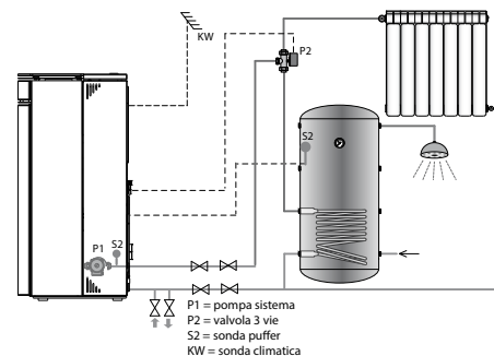
fig. 10 - Configurazione con puffer
