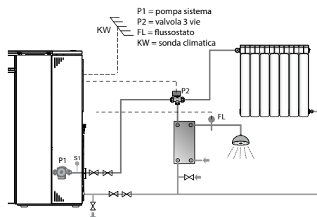
fig. 9 - Configurazione con kit sanitario
