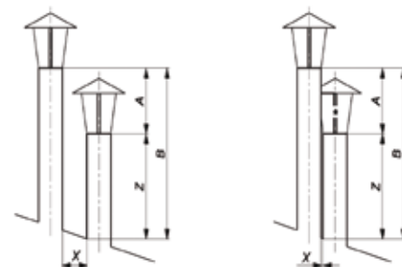
fig. 3 - Canne fumarie vicine
