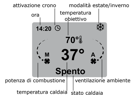
fig. 13 - Schermata principale display
