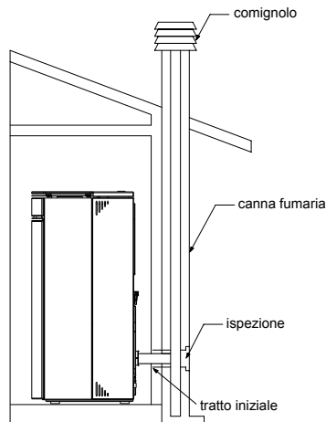
fig. 5 - Canna fumaria esistente
