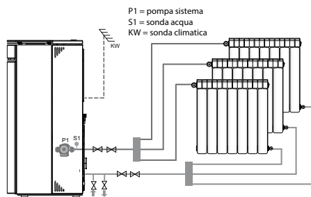
fig. 8 - Configurazione standard
