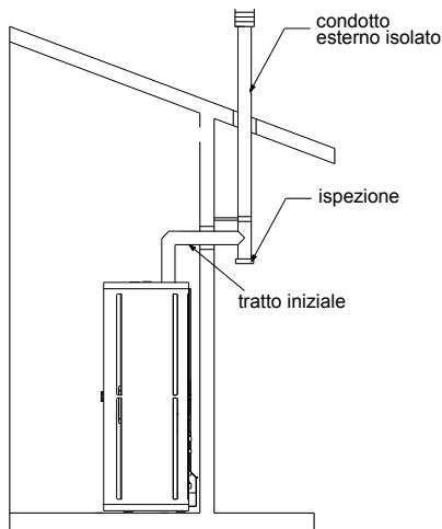
fig. 4 - Canna fumaria esterna
