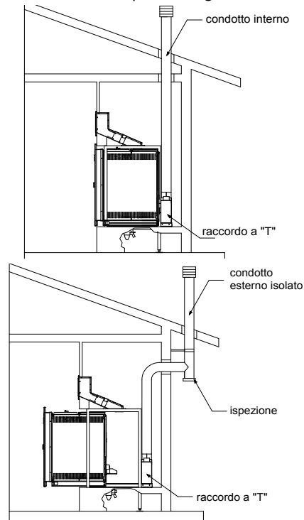
fig. 6 - Canna fumaria Yncas
