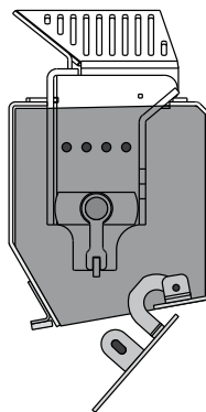
fig. 15 - Svuotamento automatico del portabraciere
