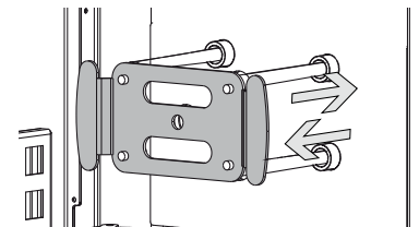
fig. 17 - Scambiatore
