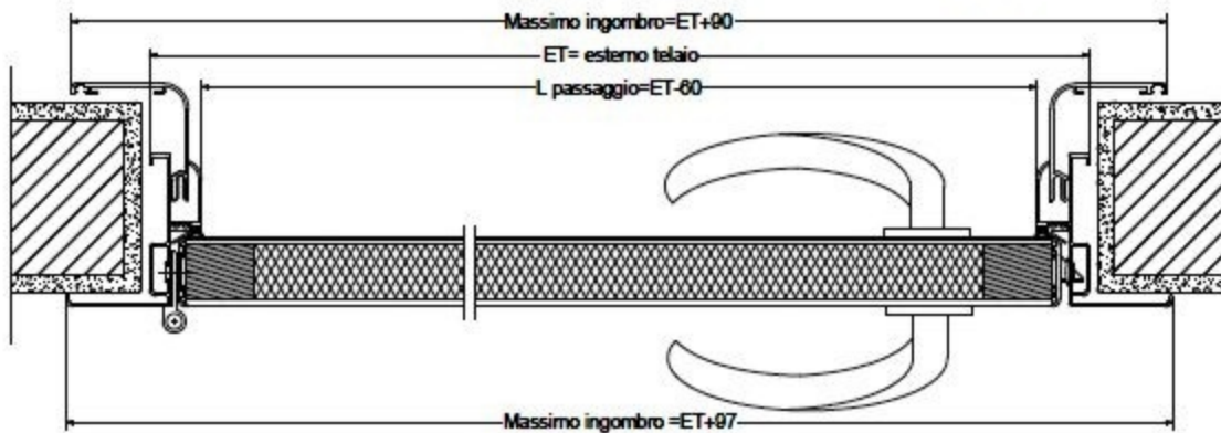
SEZIONE ORIZZONTALE
