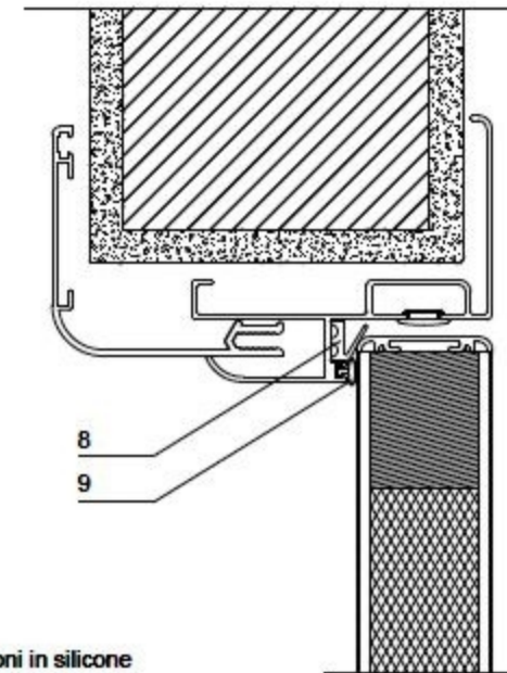
PARTICOLARE A
