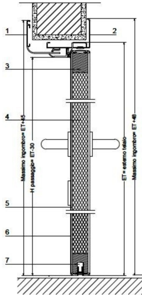
SEZIONE VERTICALE
