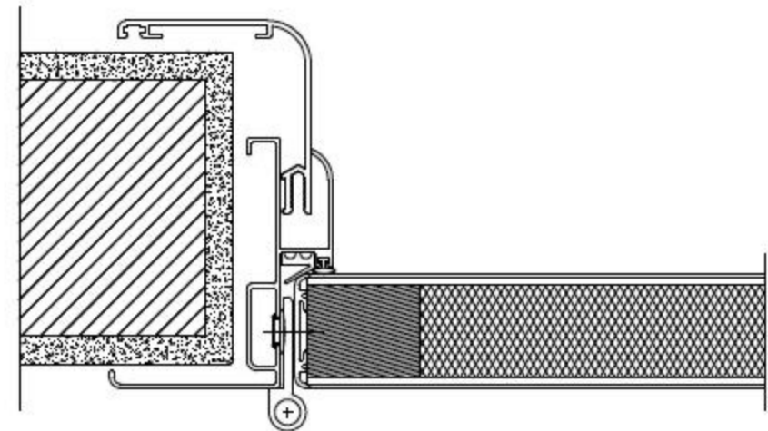
PARTICOLARE B
