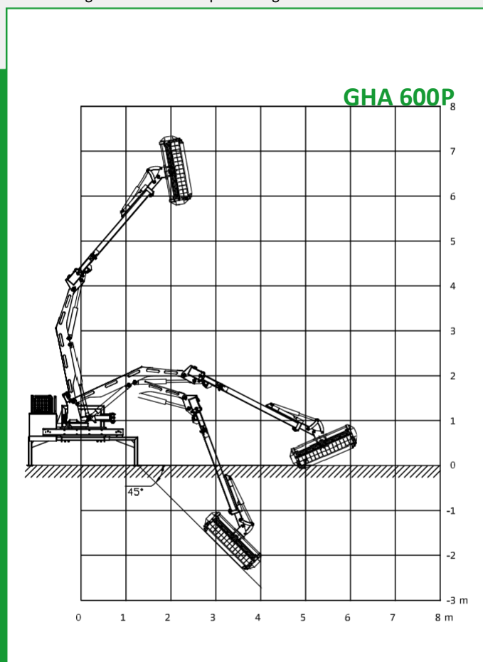
Rækkeviddediagram GHA 600 P
