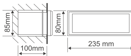
Inbouwdoo Alda
