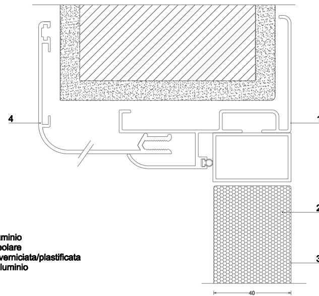
PARTICOLARE B
