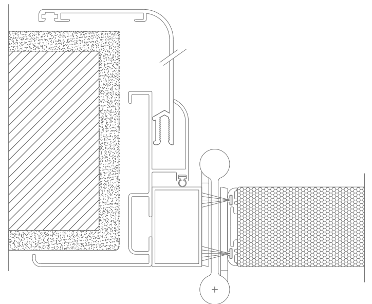
PARTICOLARE B
