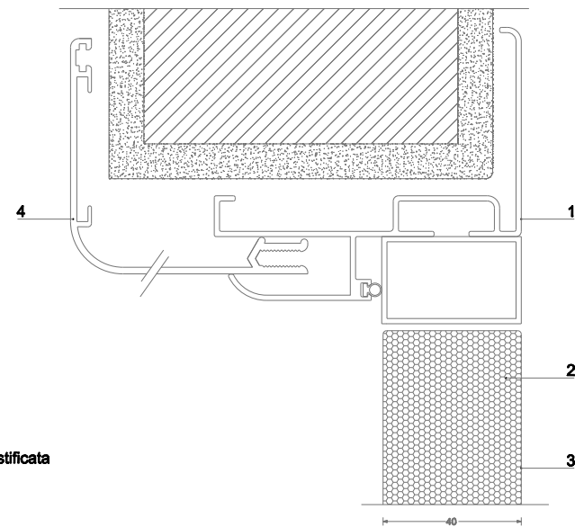
PARTICOLARE A
