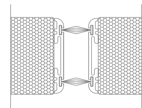
PARTICOLARE C
