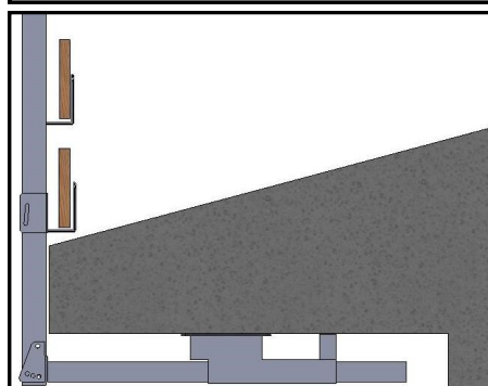
Montante installato su falda inferiore piana
