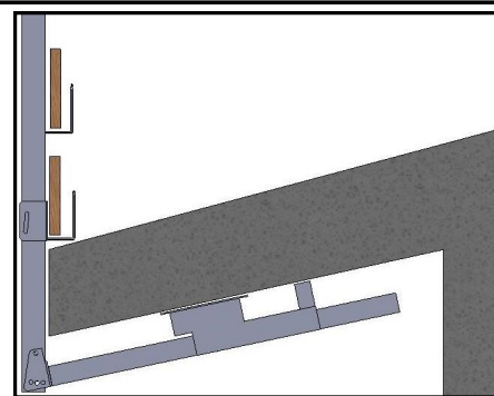
Montante installato su falda inferiore inclinata
