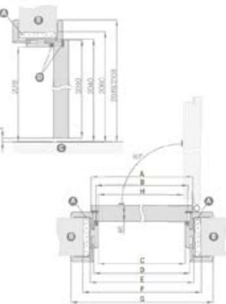
Adjustable door frame scheme
