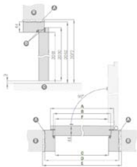
Fixed door frame scheme
