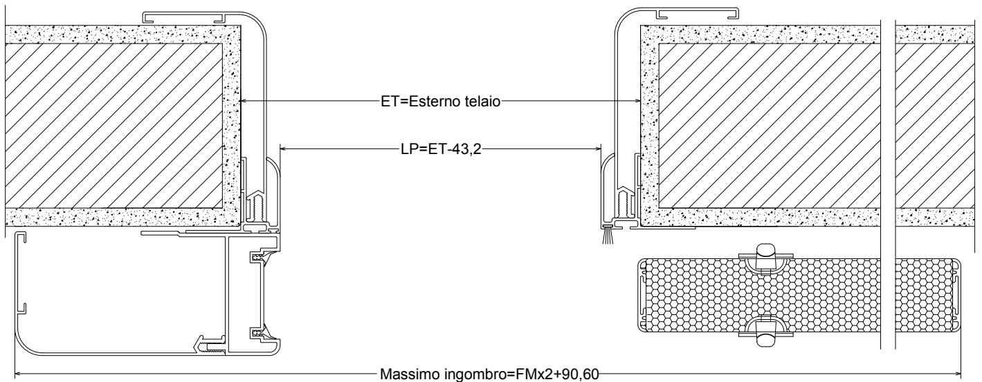
SEZIONE ORIZZONTALE
