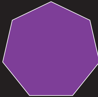
Septagon
