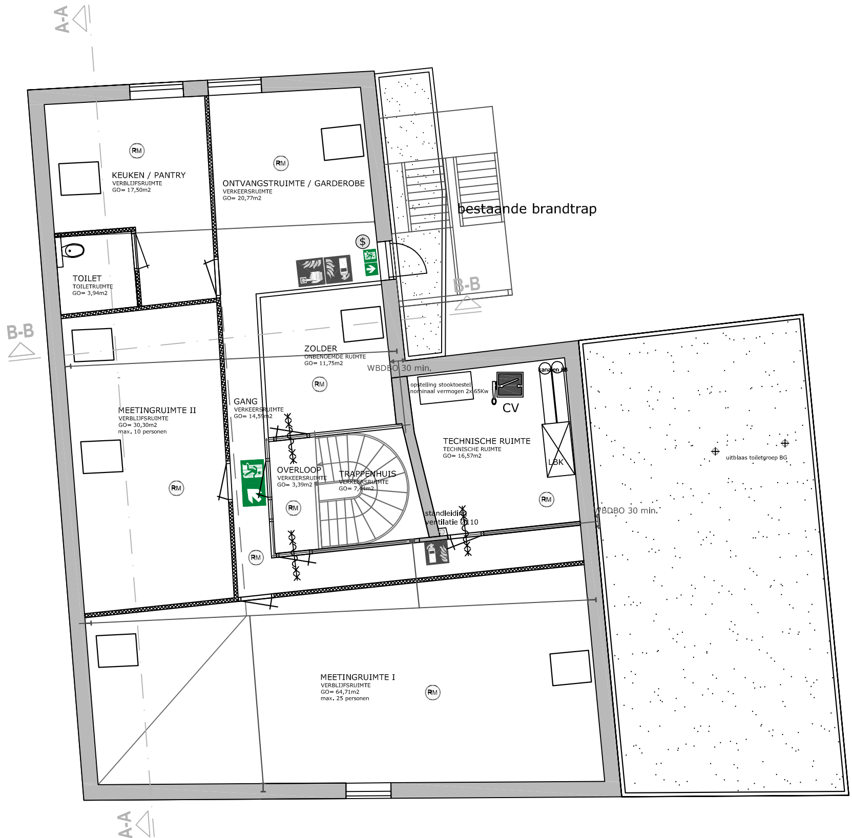
2E VERDIEPING NIEUW gebruiksoppervlak ca. 180m 2
