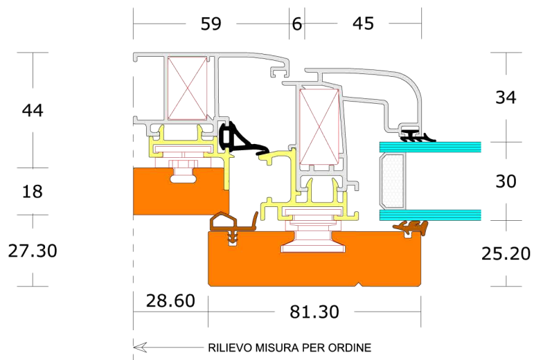
Sez. A-A: Nodo laterale telaio a Z con LRIP
