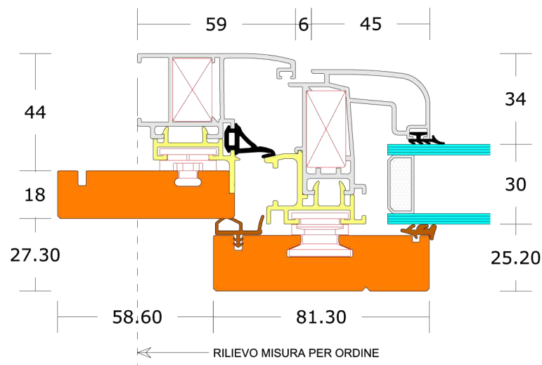
Sez. A-A: Nodo laterale telaio a Z da 30
