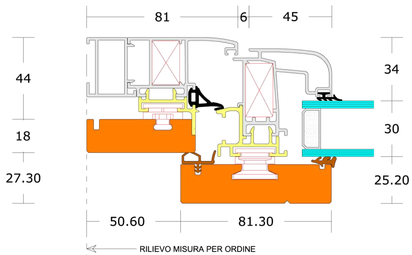
Sez. A-A: Nodo laterale telaio a Z con LRIP
