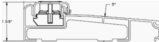
ZAA All Aluminum 3-9/16" & 4-9/16"
